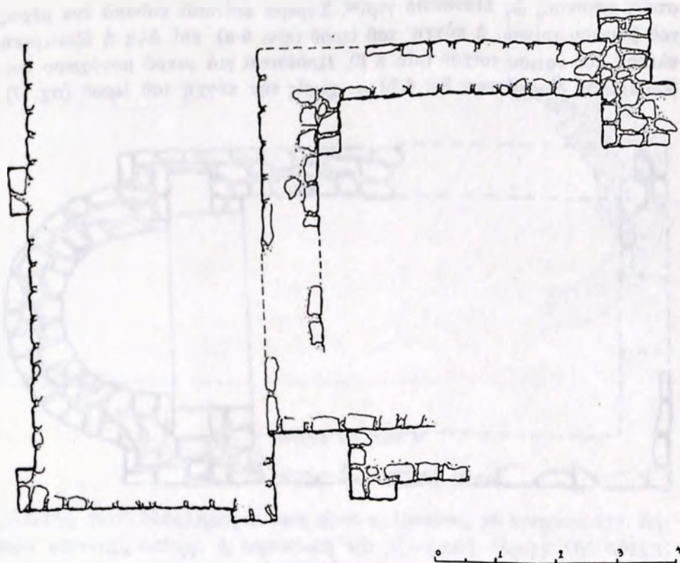
Σχ. 6. Κάτοψη του κεντρικού κτιρίου του έρειπιώνα 3.
