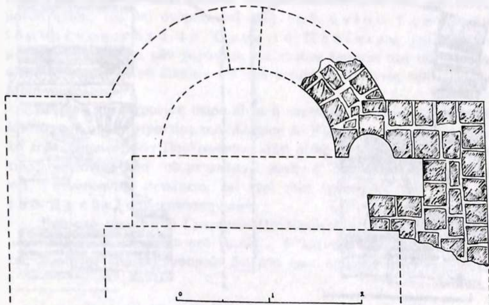
Σχ. 2. Κάτοψη του σωζόμενου τμήματος του ναού της Πελαγίας με συμπληρώσεις πού προκύπτουν άπό τά υπάρχοντα στοιχεία.
