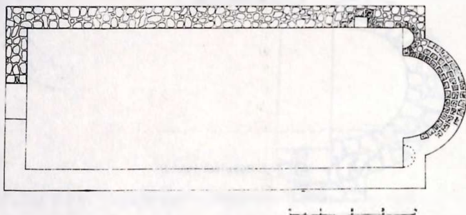
Σχ. 9. Κάτοψη τοῦ ναοῦ Γ (ἅγιος Μάριος).
