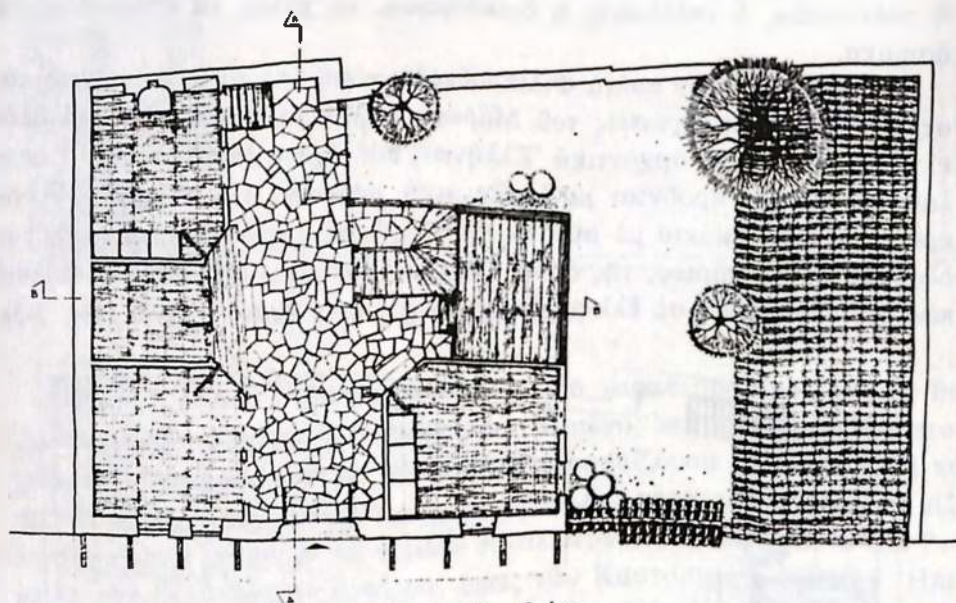
Σχ. 3. Φάση II. Ἰσόγειο.
