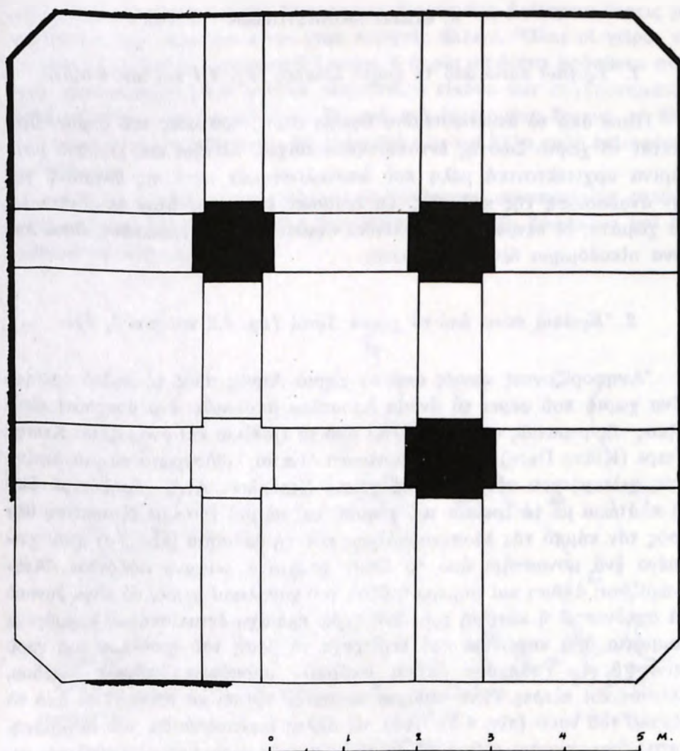
Σχ. 5. Κάτοψη τῆς κινστέρας τοῦ συγκροτήματος 2.
