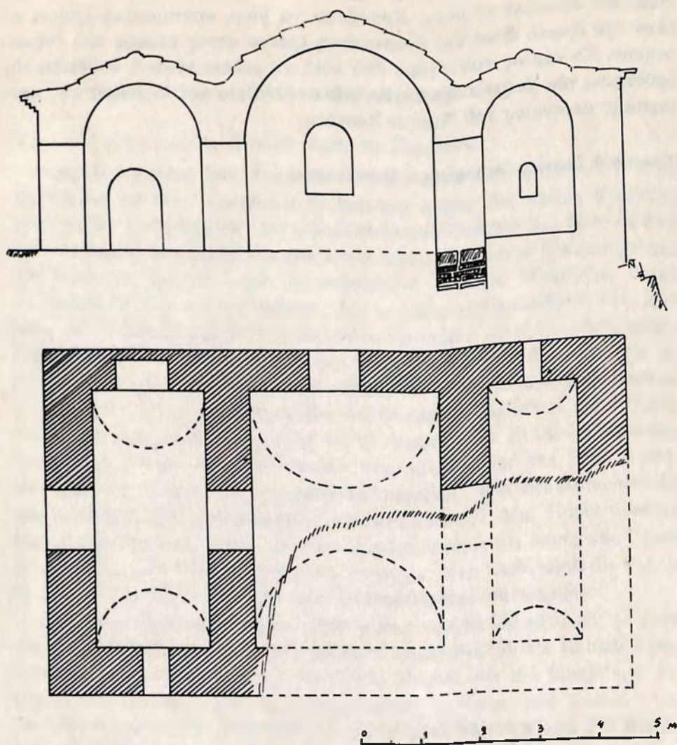
Σχ. 14. Τομή κατά μήκος και κάτοψη του μύλου στη ρεματιά Κιλισέ Ντερέ.
