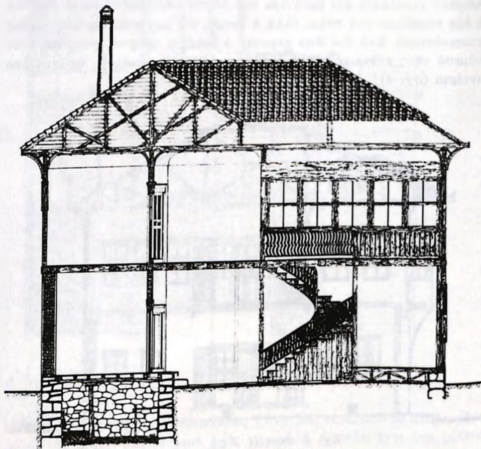
Σχ. 6. Φάση II. Τομή B-B.
