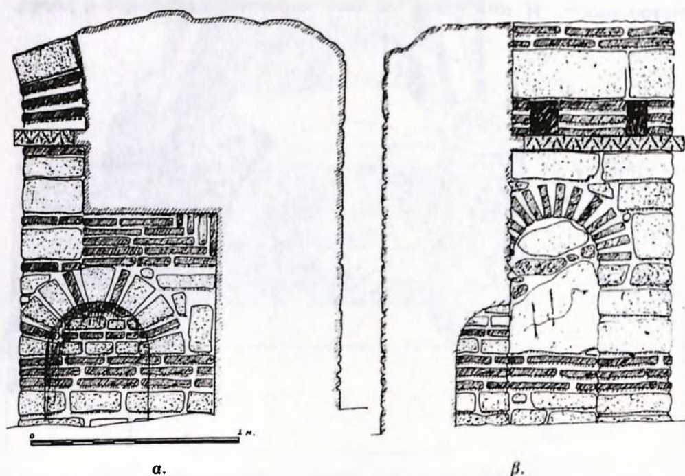
Σχ. 3. Δύο τομές της σωζόμενης ΝΑ γωνίας του ναού της Πελαγίας. Προβολή τών στοιχείων της έσωτερικής παρειάς του ανατολικού τοίχου (α) και του νότιου τοίχου (β).
