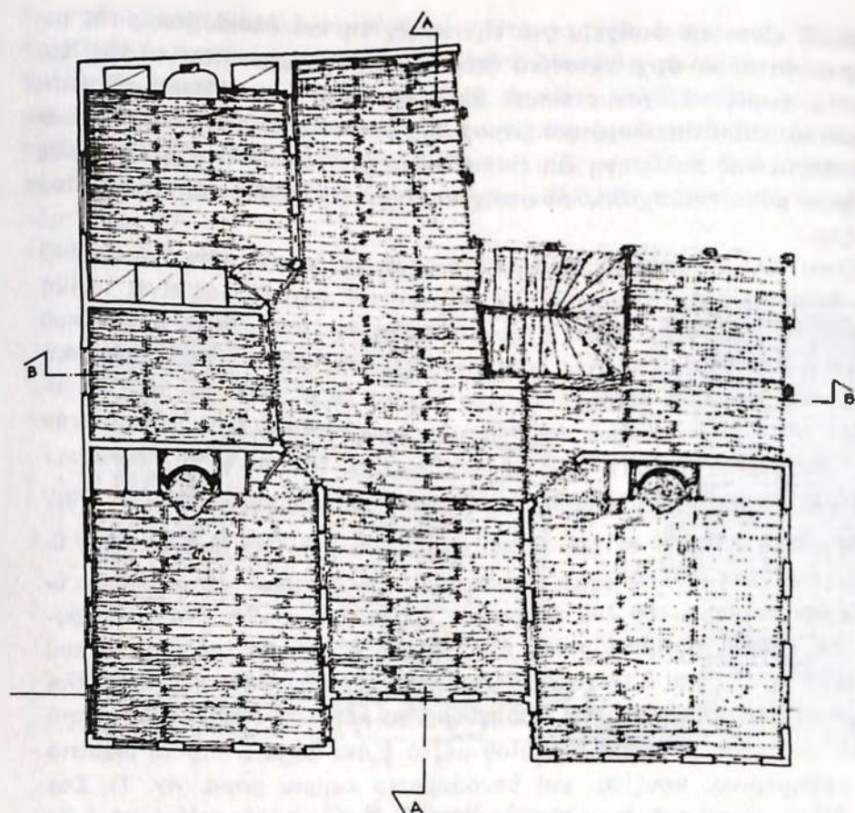
Σχ. 4. Φάση II. Όροφος.
