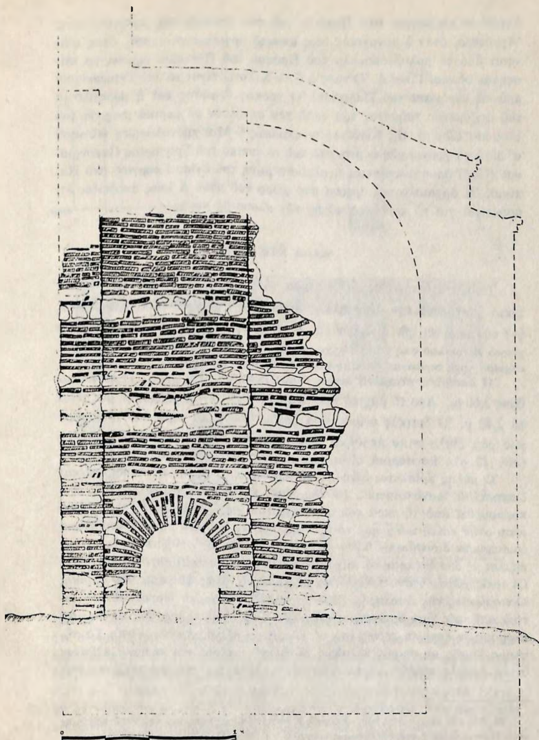
Σχ. 13. Τομή κατά μήκος του Ιεραῦ. Μερική ἀποκατάσταση.
