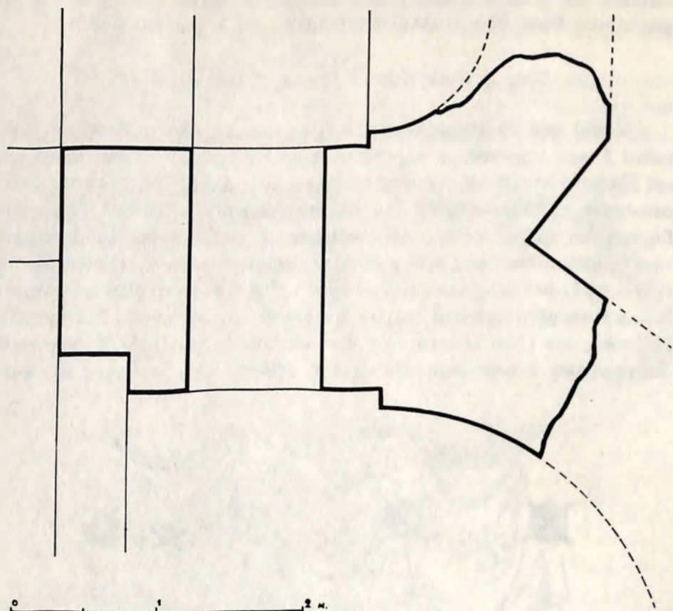
Σχ. 11. Κάτοψη του ορατού τμήματος του ναού Δ ("Ακ Κιλισέ).
